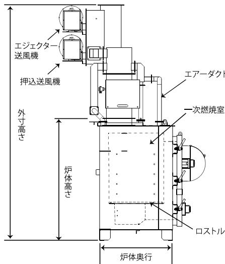
側面図
