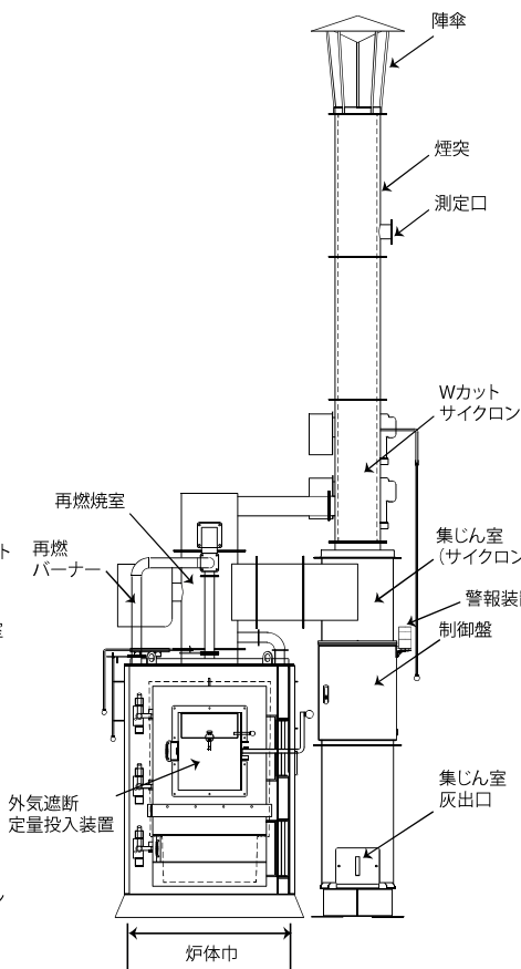
正面図
