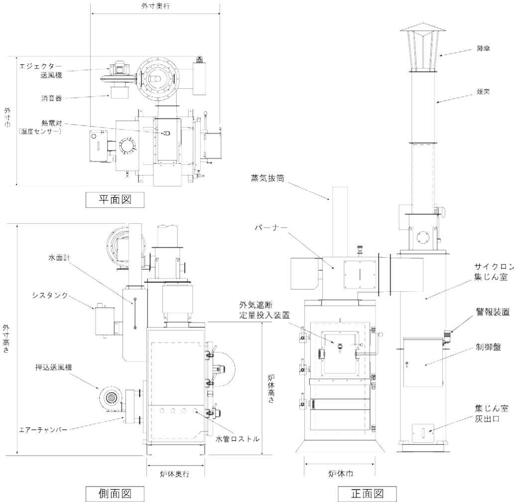
図面はISR-500M
